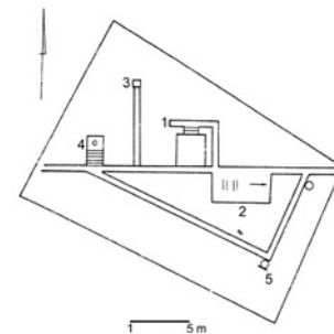
Ryc. 51 – Rozmieszczenie przyrządów w ogródku meteorologicznym
